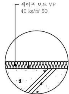
"C" 부분상세도
