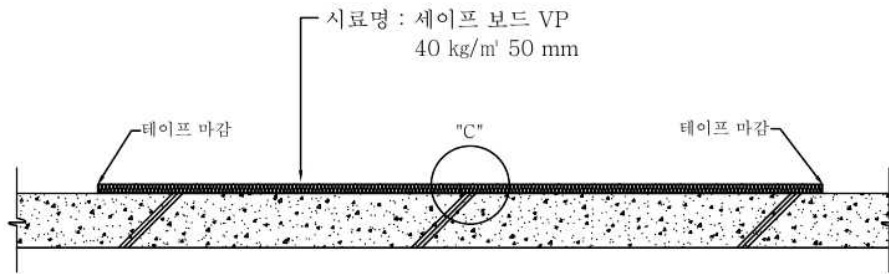
B-B' 단면도
