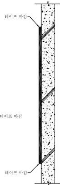
A-A' 단면도
