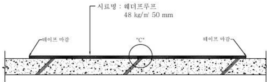
B-B' 단면도
