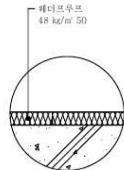
"C" 부분상세도
